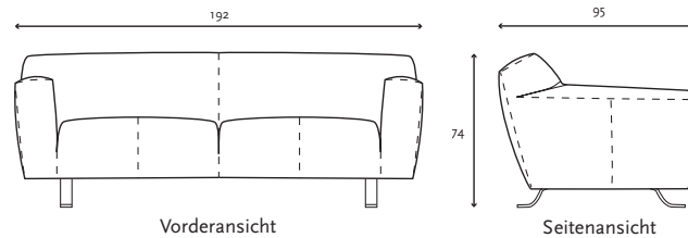
Vorderansicht
